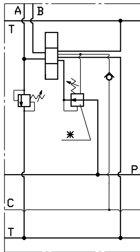
Исполнение 1- с предохранительным клапаном в гидролинии А
